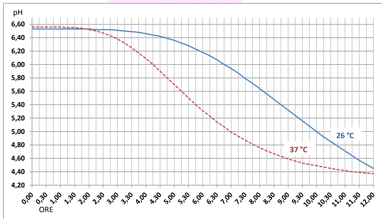
CURVA ACIDIFICAZIONE
